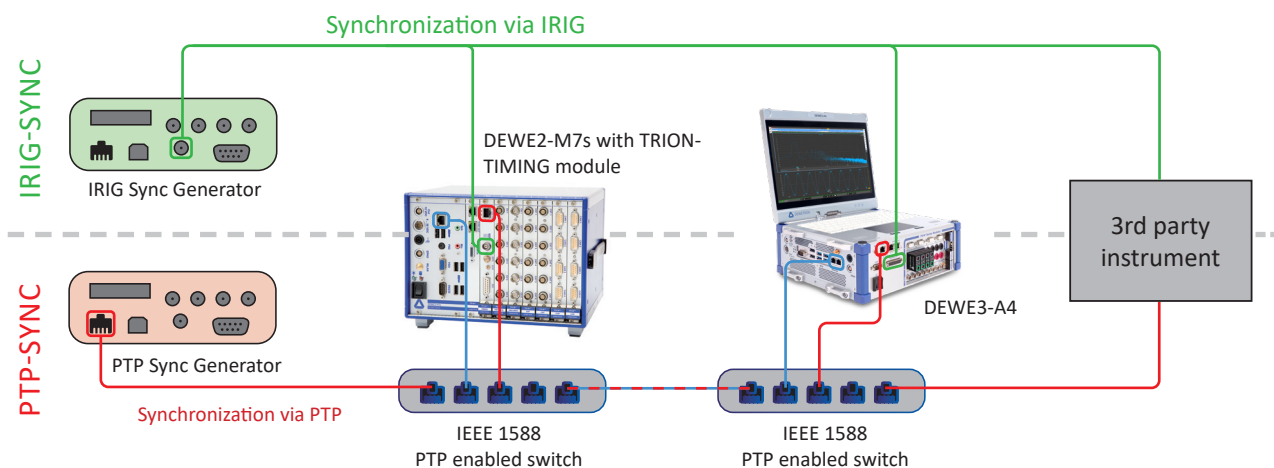
Fig. 25: PTP sync / IRIG sync
